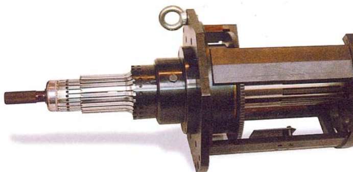
Insertadora semi-automática ISV-200 Semiautomatic inserting machine ISV-200
