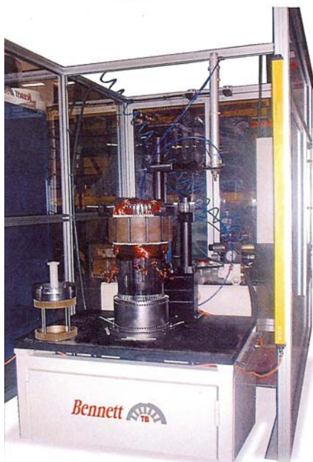
Insertador alternadores Inserting tool alternator
